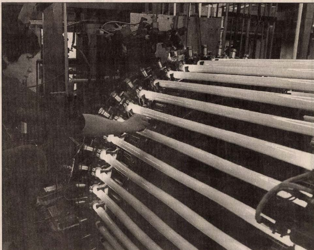
A fénycsőgyártó gépsor
